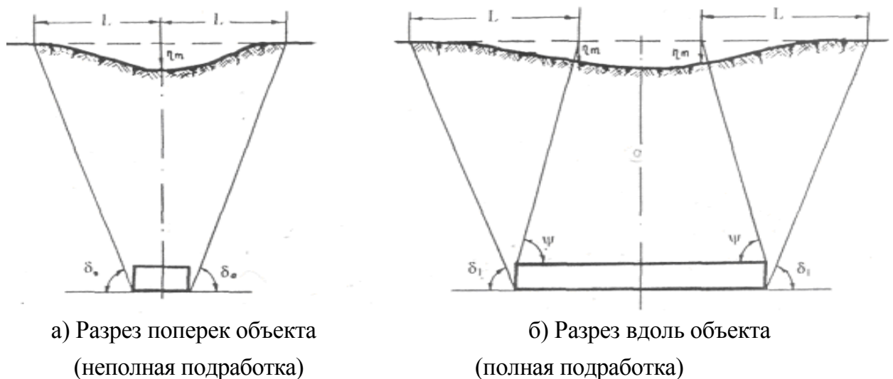
Р и с у н о к С.1 - Основные параметры мульды сдвижения
